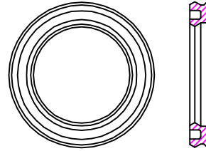
3 PC VHPC-2210 (ROD SEAL)
